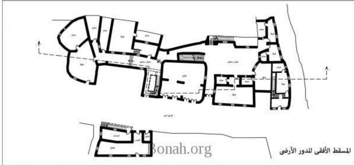
الشكل (10), المسقط الافقي للدور الارضي البابنشال, واحة سيوة.
